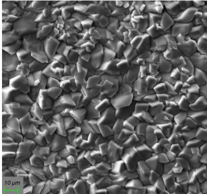
SURFACOTE MN 2, 500fache Vergrößerung
