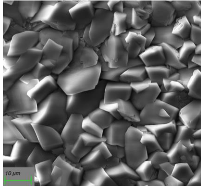
SURFACOTE MN 2, 1000fache Vergrößerung
