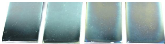
AZUR HT4 + PROSEAL CF 330 nach 96 h im Salzsprühtest nach DIN EN ISO 9227
