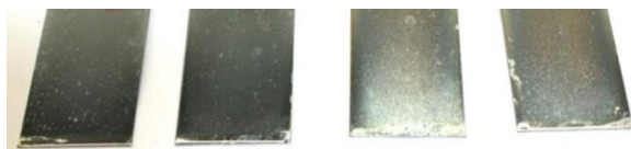
AZUR HT4 + PROSEAL CF 330 nach 240 h im Salzsprühtest nach DIN EN ISO 9227
