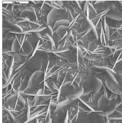
SURFACOTE 125, 1000fache Vergrößerung
