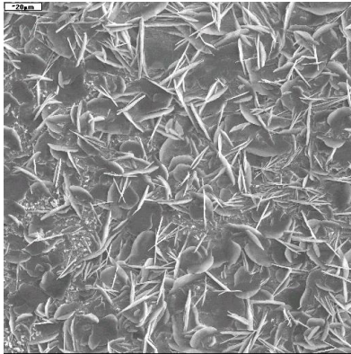
SURFACOTE 125, 500fache Vergrößerung
