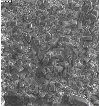
SURFACOTE MN 2, 500fache Vergrößerung
